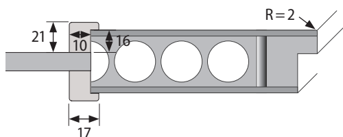
QUERSCHNITT TÜRLATT | GLASLEISTE
